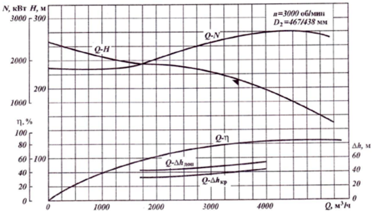
Рисунок А.12 – Рабочая характеристика насоса НМ 7000-210 со сменным ротором на подачу 3500 \text{ м}^3/\text{ч}
