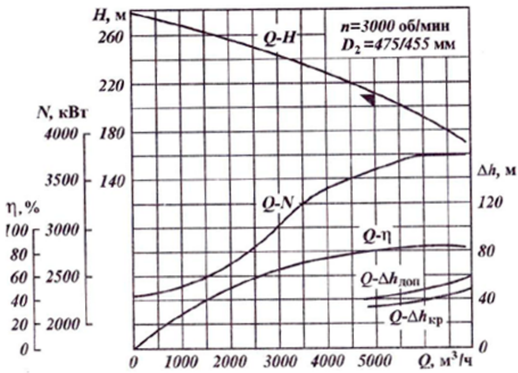
Рисунок А.15 – Рабочая характеристика насоса НМ 10000-210 со сменным ротором на подачу 5000 м³/ч
