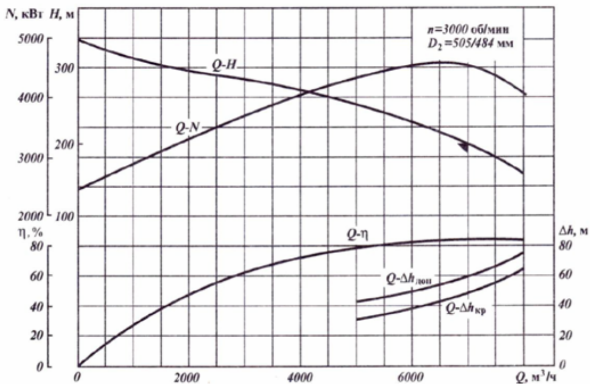
Рисунок А.16 – Рабочая характеристика насоса НМ 10000-210 со сменным ротором на подачу 7000 м³/ч
