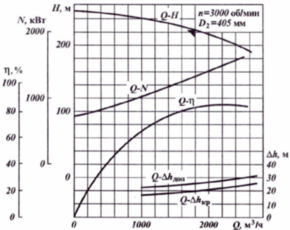
Рисунок А.4 – Характеристика насоса НМ 2500-230 со сменным ротором на подачу 1800 \text{ м}^3/\text{ч}
