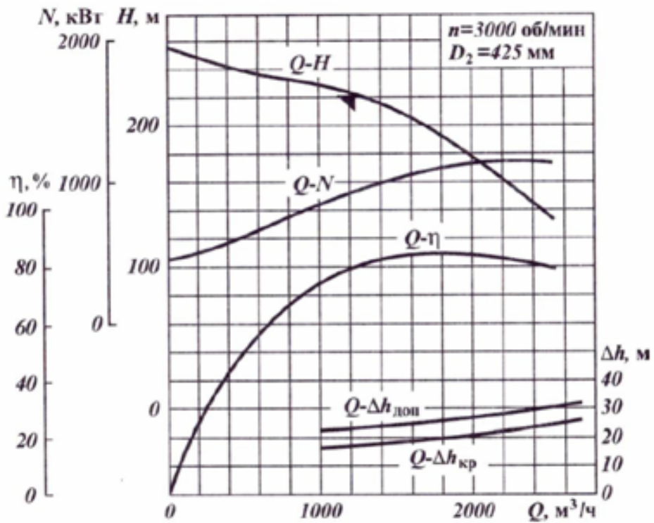
Рисунок А.3 – Характеристика насоса НМ 2500-230 со сменным ротором на подачу 1250 \text{ м}^3/\text{ч}
