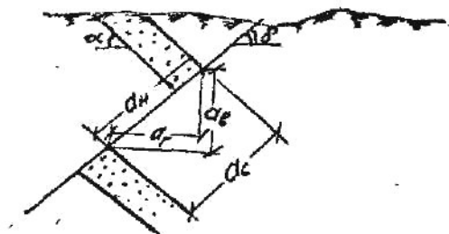
Рис. 3.5. Взброс и его элементы: a_c, a_v, a_g, a_n – амплитуды смещения (см. рис. 3.4), \alpha – угол наклона пласта, \delta – угол наклона сместителя, a_g – горизонтальная амплитуда смещения взброса или перекрытие (сдвигание).
