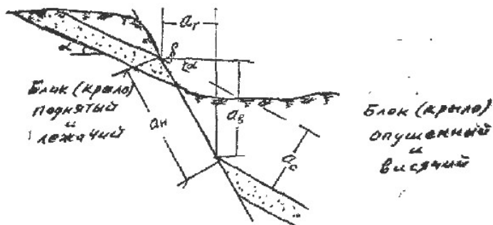
Рис. 3.4. Нормальный (согласный) сброс и его элементы: a_c, a_v, a_g, a_n – амплитуды смещения; a_c – стратиграфическое, a_v – вертикальное, a_g – горизонтальное (зияние), a_n – наклонное (по сместителю), \alpha – угол наклона пласта, \delta – угол наклона сместителя.
