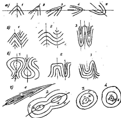
Рис. 3.2. Морфологические типы складок в разрезе – а, б, в и в плане – г : а) 1 – прямая, 2 – наклонная (косая), 3 – опрокинутая, 4 – лежачая, 5 – перевернутый антиклиналь; б) 1 – открытая остроугольная, 2 – открытая обычная, 3 – изоклиальная; в) 1 – веерообразная, 2 – сундучная (коробчатая) с широкими плоскими замками и крутыми крыльями: гребневидные (3) (антиклинали) и килевидные (2) (синклинали) между сундучными складками; г) 1 – линейная, 2 – брахискладка, 3 – купол, 4 – чаша.
