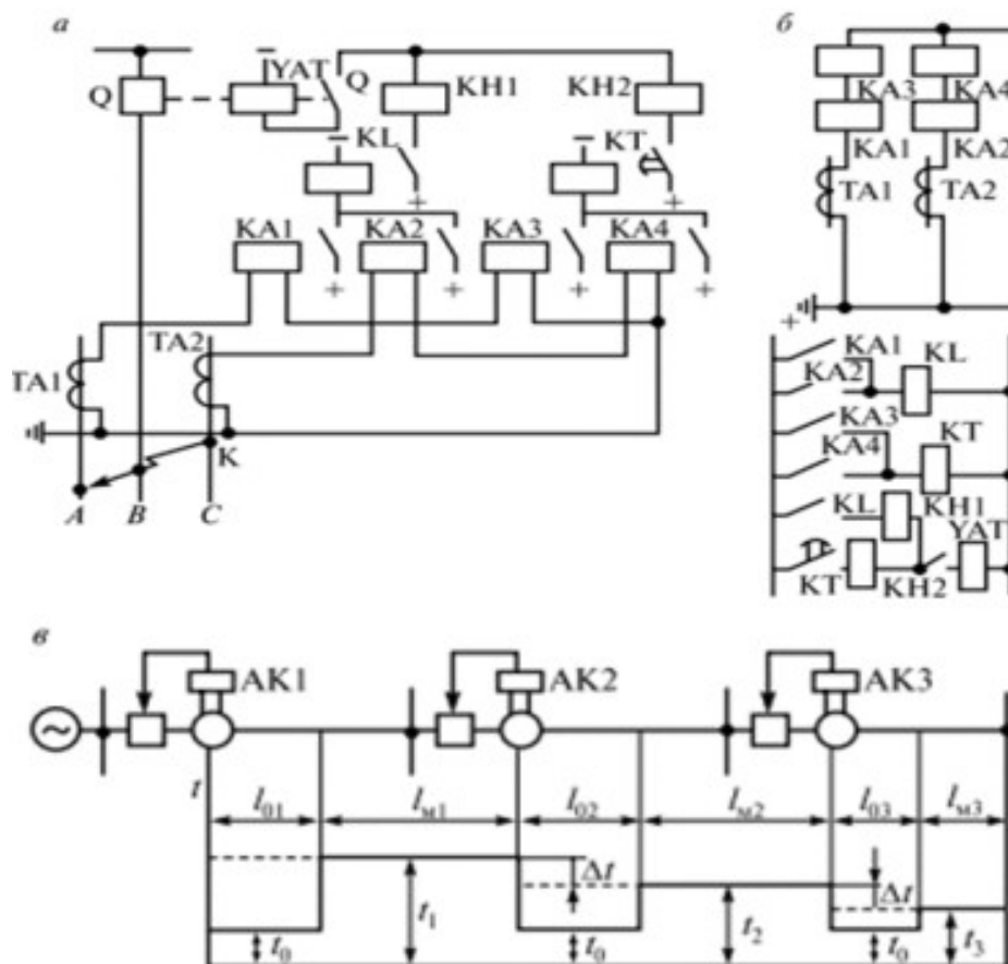
Рис. 2.1. Комбинированная схем защиты МТЗ и ТО: а) совмещенная; б) разнесённая; в) диаграмма времени срабатывания защит
