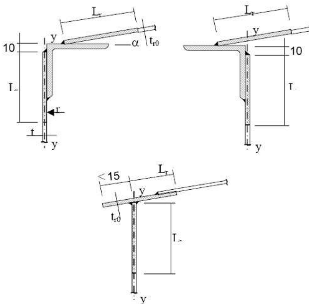
Рисунок 2 – Соединения конической крыши со стенкой
