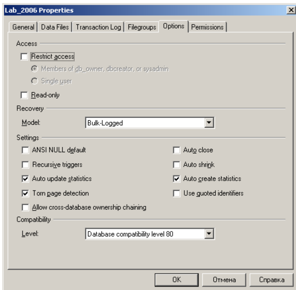
Рис 3.5. Вкладка OPTIONS
