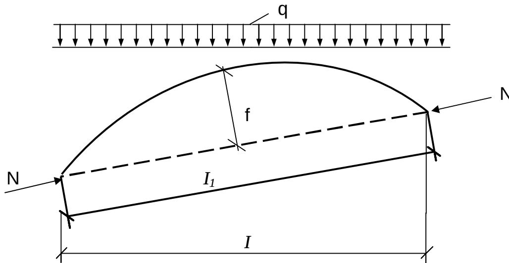
Рис. 5.7. Расчётная схема панели верхнего пояса сегментной фермы
