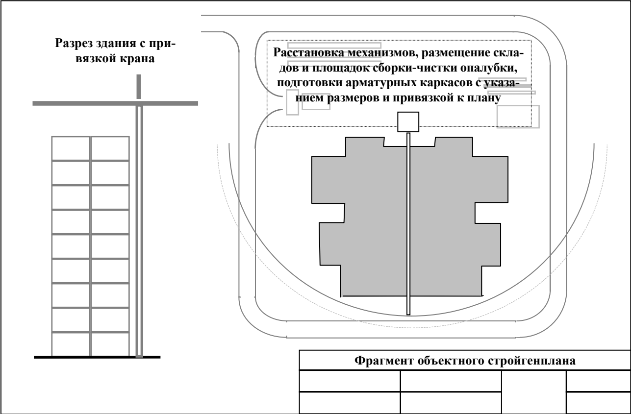
Рис. 5. Примерная компоновка графических листов формата А3 при оформлении решений по стройгенплану и календарному плану работ на объекте
